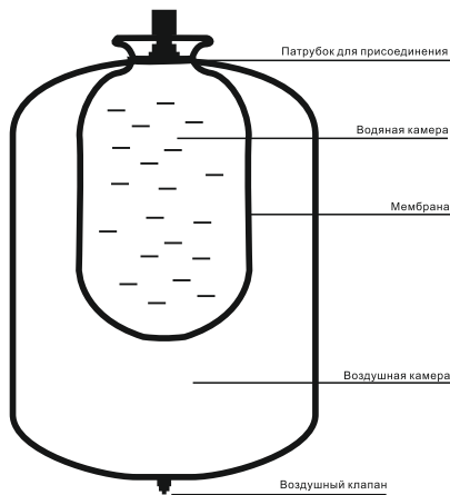
Рис. 1. Конструкция бака
